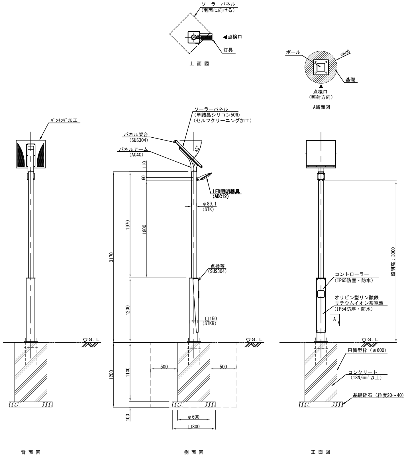
ソーラー照明 (ST5014R3) 姿図 S=1:40 (ストークスタンダード)
