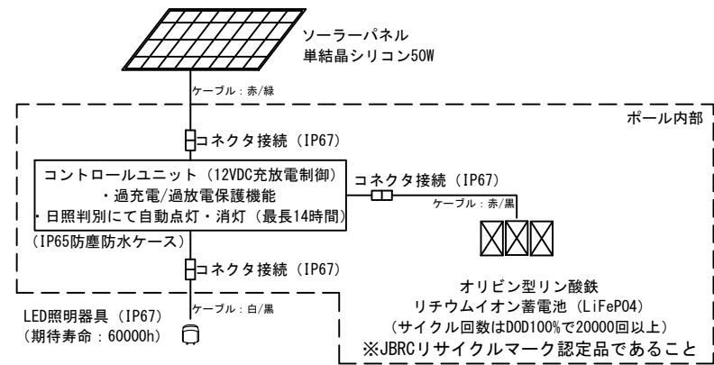
システム系統図・結線図
