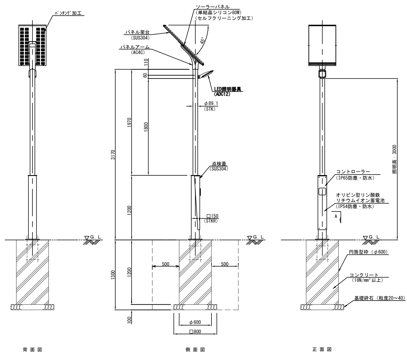
ソーラー照明 (STJ8014R4) 姿図 S=1:40 (ストック和風)
