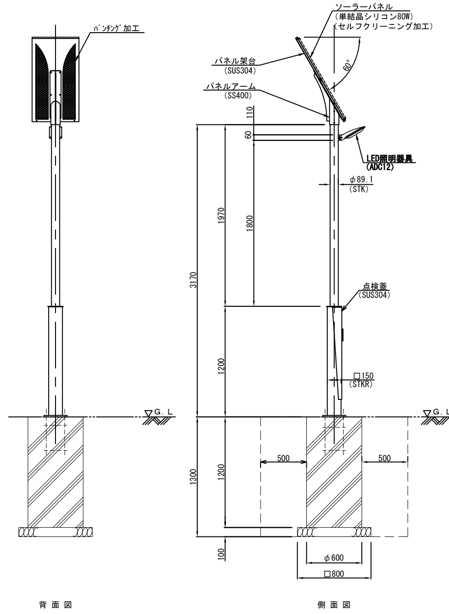
ソーラー照明 (STS8014R4) 姿図 S=1:40 (ストック積雪地域対応型)
