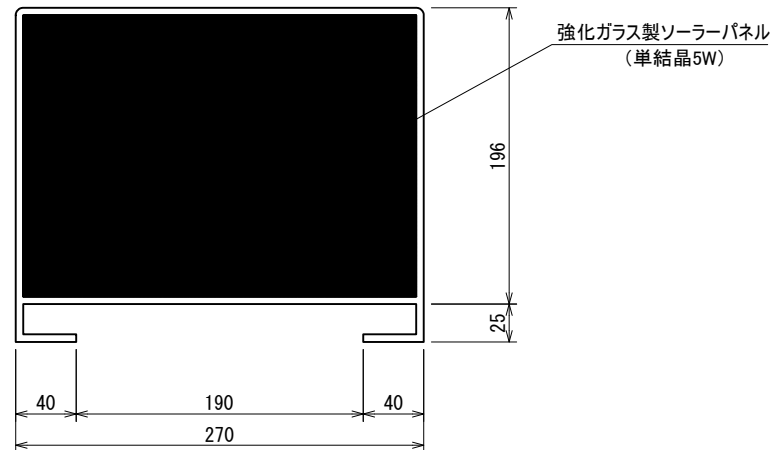
上面図
