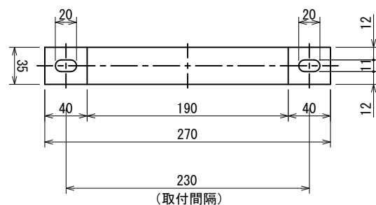
背面図
