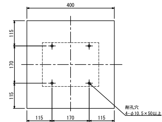
基礎天端図
