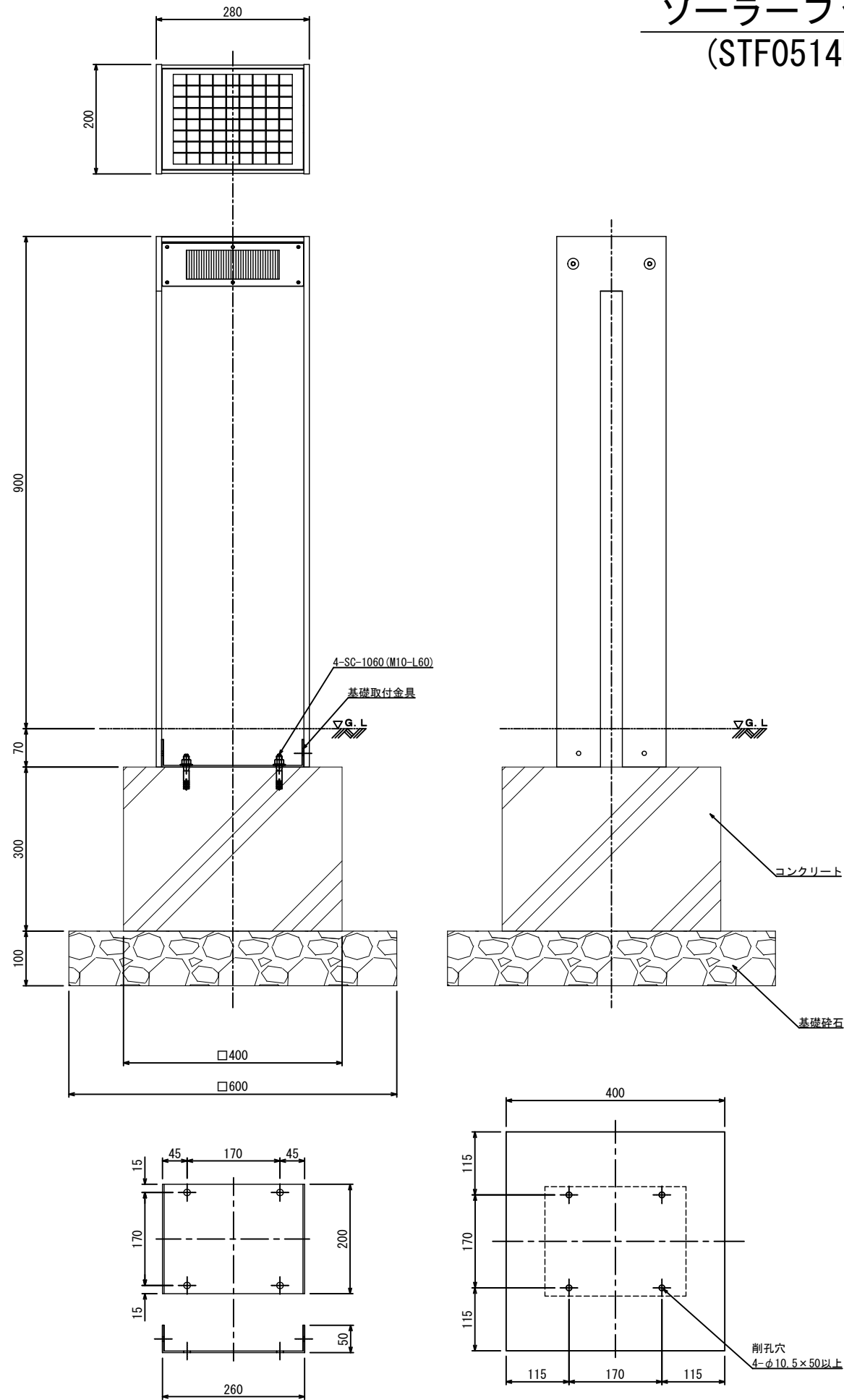
基礎取付金具詳細図
