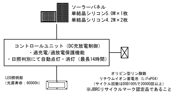
システム系統図
