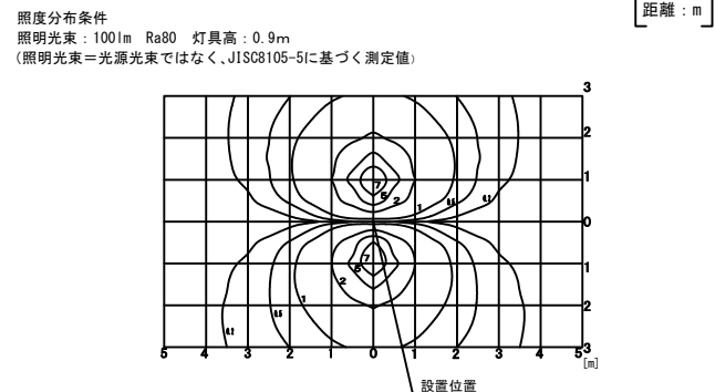
水平面照度分布図
